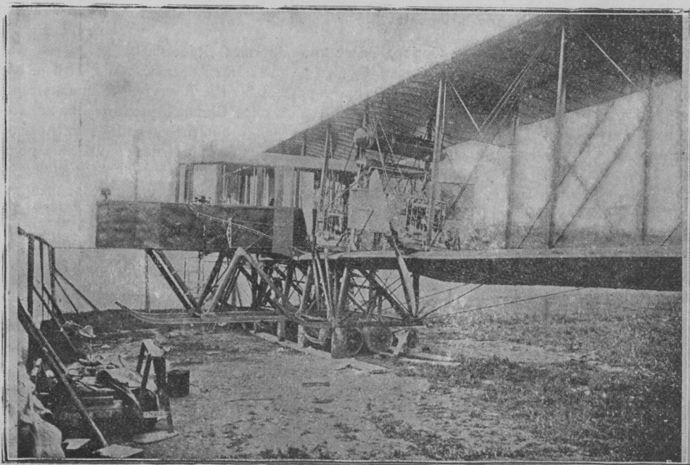
Aeroplan-omnibus, s katerim se more dvigniti 10–15 vojakov v zrak, da opazujejo ali obstreljuje sovražnikovo kretanje.
