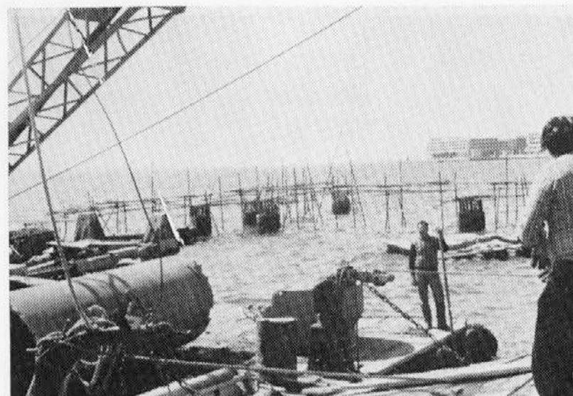
Začetek gradnje pomola za skladiščem soli v Portorožu
