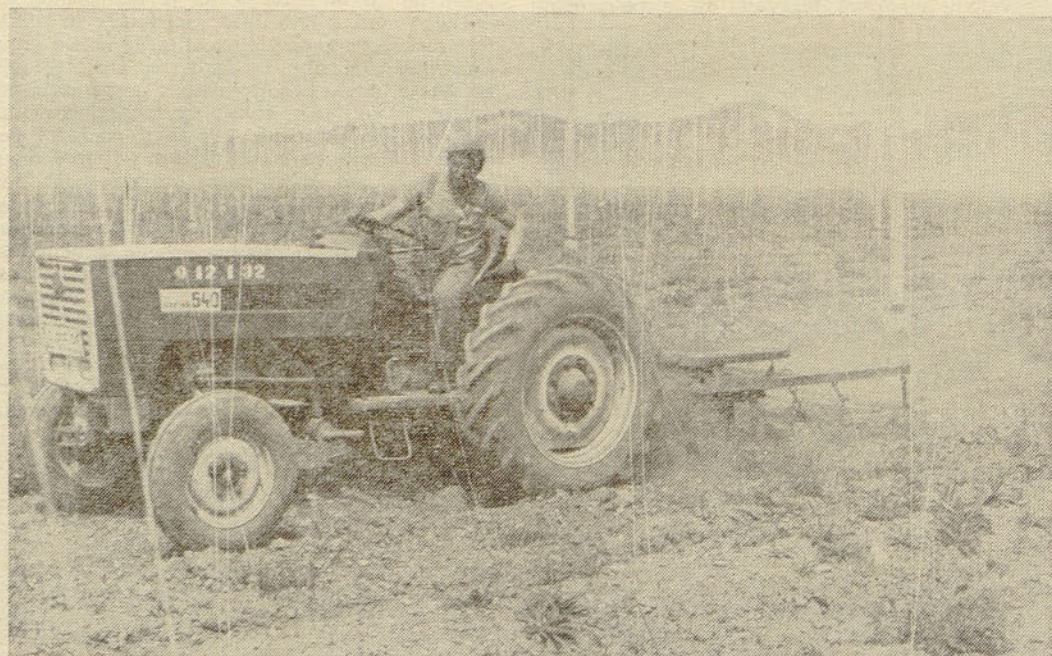
— Prvo rahljanje zemlje po napeljavi vodil je zahtevno in pomembno opravilo. V prerahljano zemljo zamešamo gnojila in uničujemo plevela, mislimo pa tudi že na varčevanje z vlago. Kultivatorju pripeta brana izboljša kvaliteto dela.
