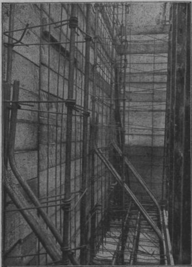
Zseleznoga betona sztena pri tórmí szobocske cérkvi.
