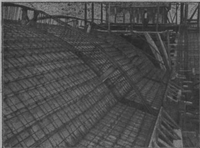
Narejeno zselezo za beton pri velkih dverah szobocske cérkvi.
