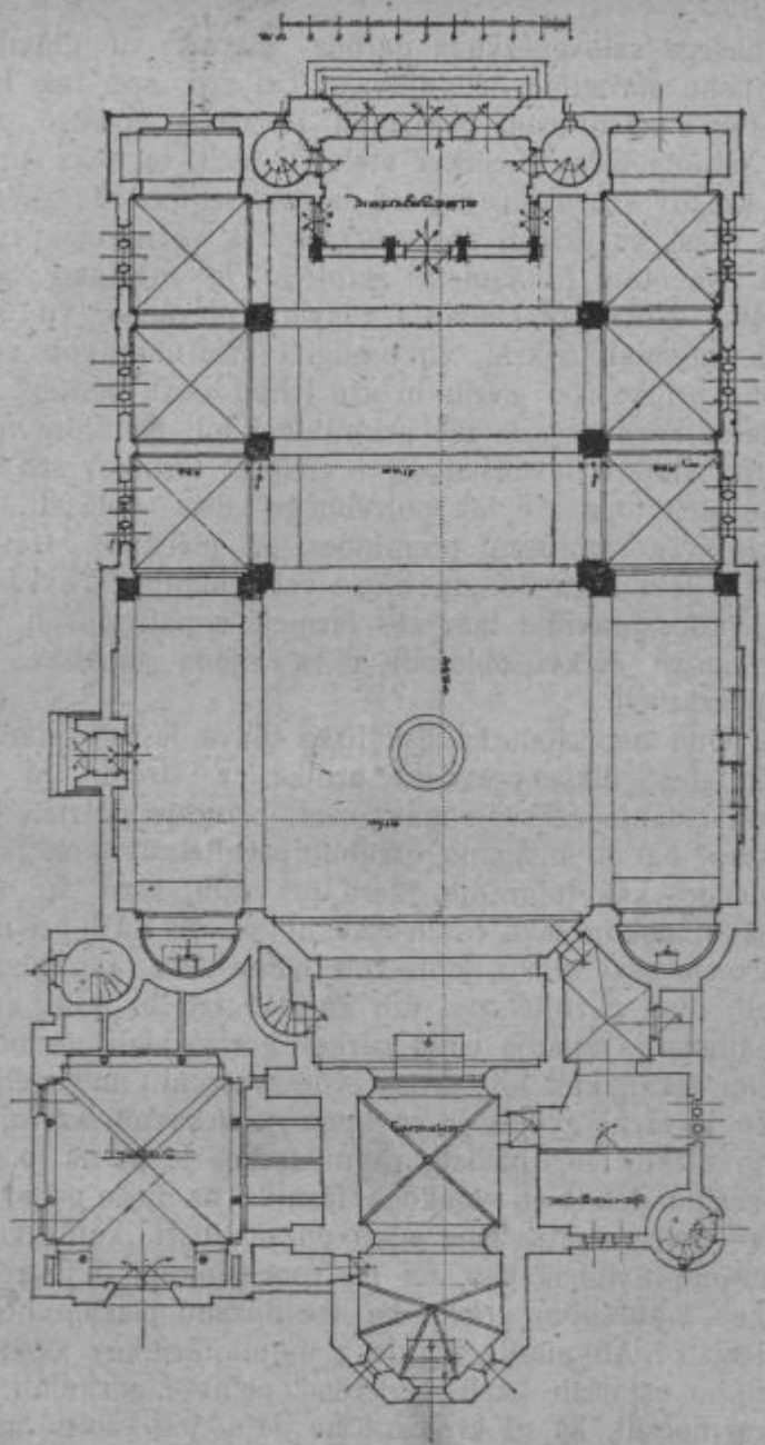
Fundamentální risz szobocské cirkvi.
