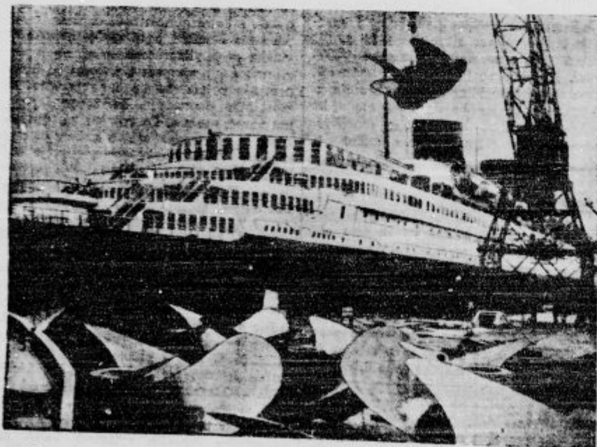
francoske veleladje Normandis popravljajo, ker : hočejo dati večjo hitrost. Pritrjujejo ji nove, nekoliko lažje vsake, ki tehtajo le po 22 ton vsak.
