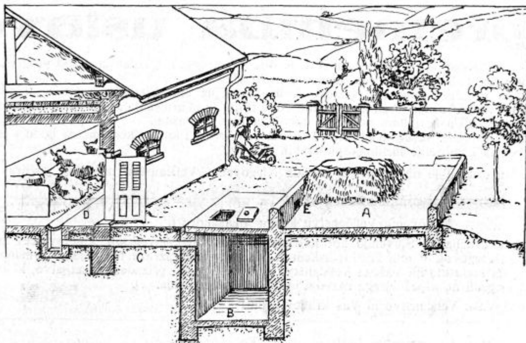
Slika 1. Pogled na hlev, gnojišče in gnojnično jamo od zgoraj in v prerezu. A gnojišče, B gnojnična jama, C gnojnični jarek, D gnojnični žleb, E luknja za odtekanje gnojnice izpod gnoja v gnojnično jamo.
