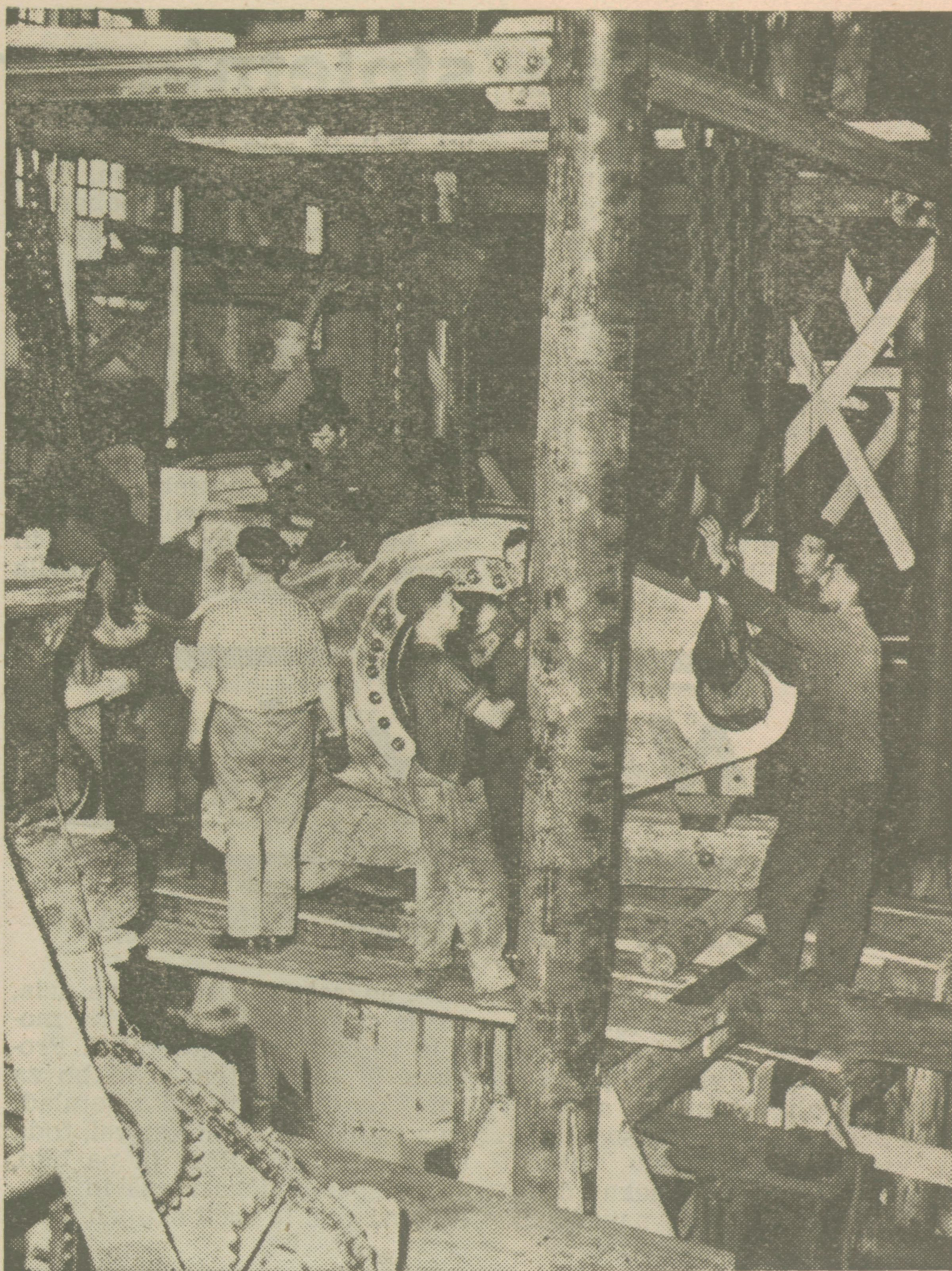
Eden od treh cilindrov pri montaži Foto H. Poročnik
