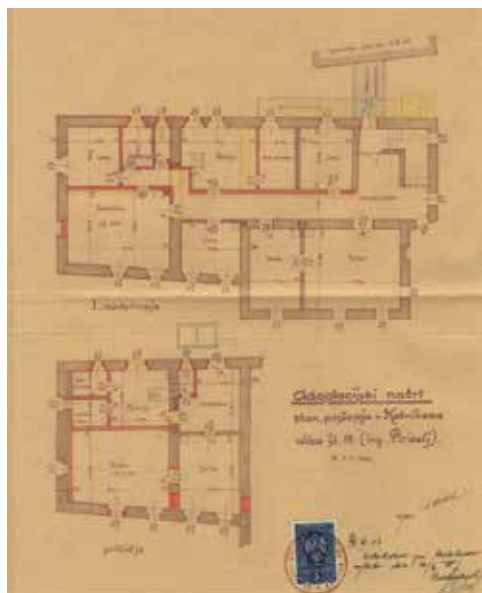
Preureditveni načrt hiše Josipa Briclja ml., 1935 (ZAL, VRH 2).
