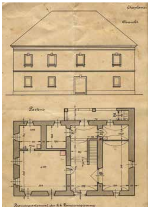
Načrt za prenovu kaplanije, 1909 (NŠAL, ŽA Vrhnika).
