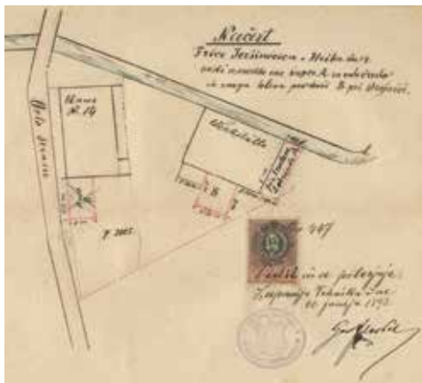
Načrt za gospodarsko poslopje in hlev pri usnjarni Friderika Jeršinovica, 1893 (ZAL, VRH 2).
