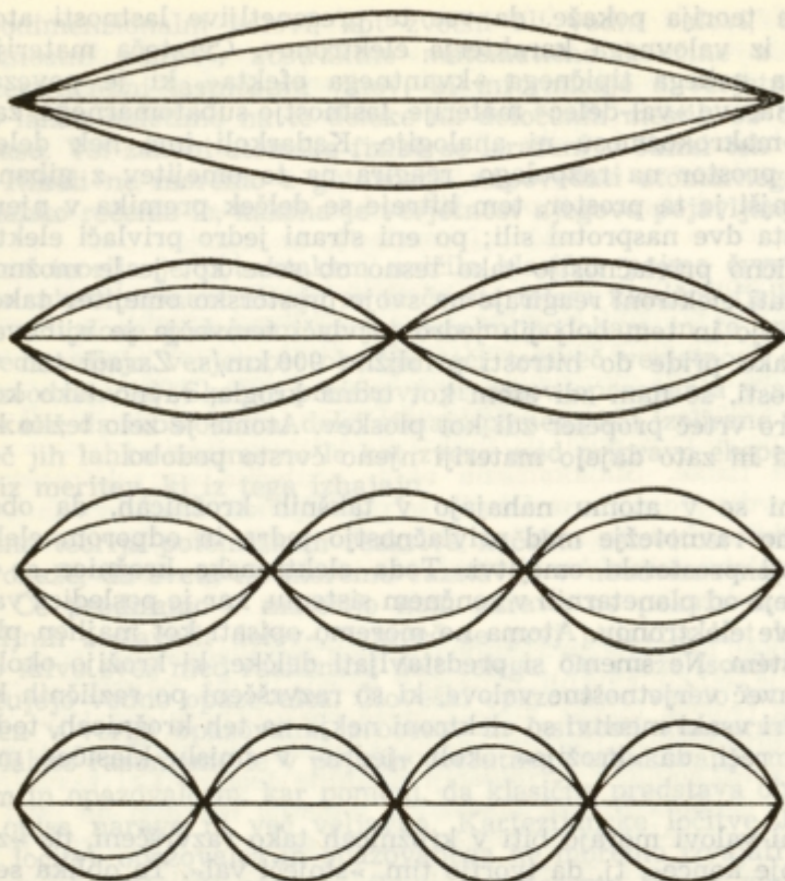
stoječi val nihajoče strune
