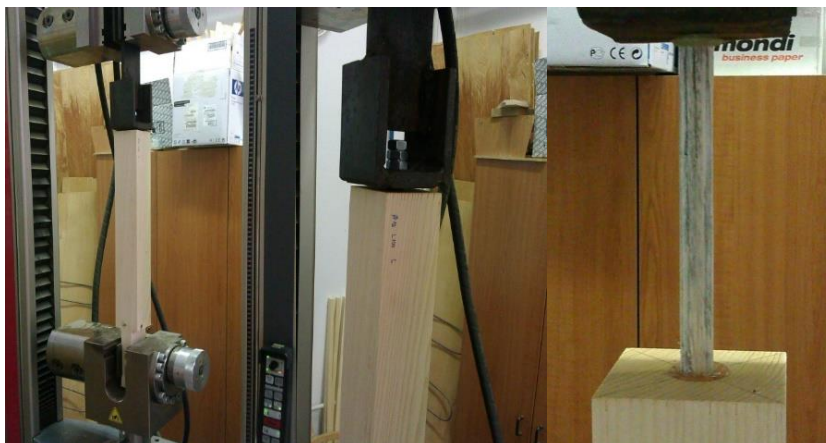
Slika 3. Vpetje VIVJP v univerzalni testirni stroj Zwick Z100 (levo), detajl vpetja vijaka z metričnim navojem (v sredini) in porušitev VIVJP preskušanca po lesnih vlaknih (desno).
