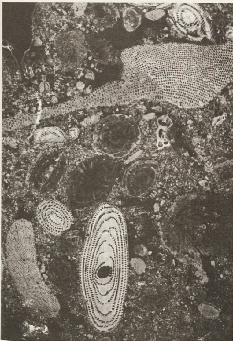
Alveolinsko-numulitni apnenec; zbrusek je povečan, v naravni velikosti je širok 1 cm! foto: M.Grm
