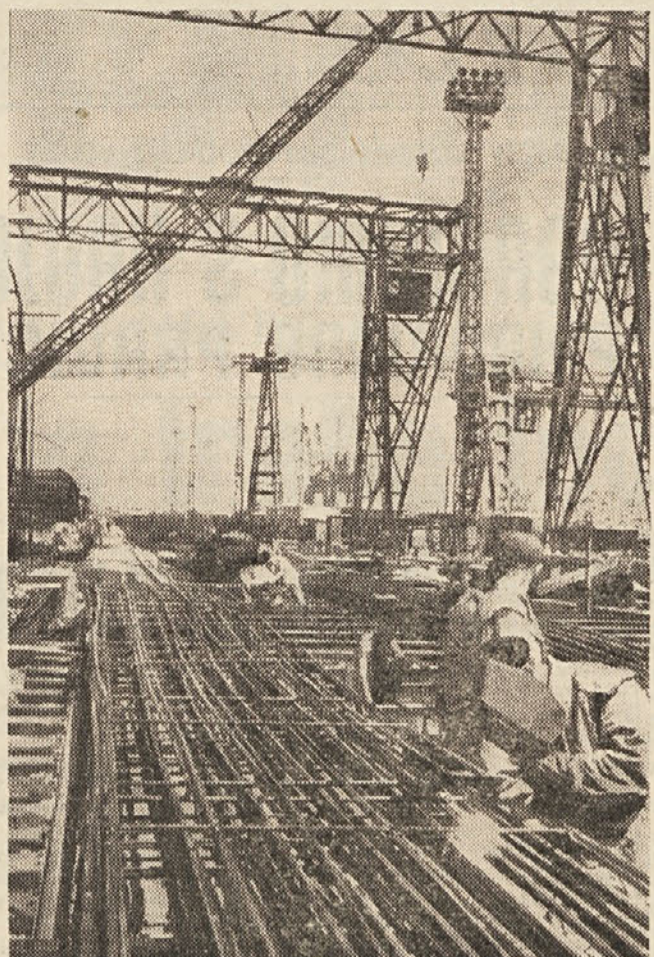
Velikanske delavnice v Kujbiševu, v katerih pripravljajo železno ogrodje za betonsko gradnjo
