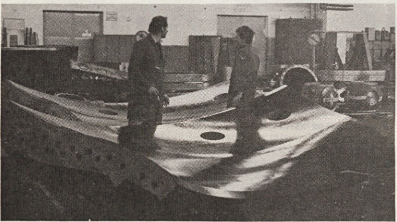
Šestdelni zunanji vodilnikov obroč za cevno turbino HE Dubrava. Deli so v fazi površinske zaščite pred poskusno montažo. V delavnici bo vodilnik sestavljen in funkcionalno preizkušen in kot sklop v dveh delih prepeljan
