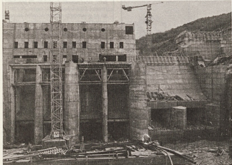
Izstopni del centrale z delom bodoče upravne stavbe
