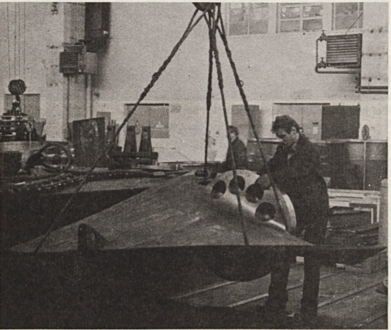
Prve lopate za gonilnik. Transport med vmesnimi operacijami
