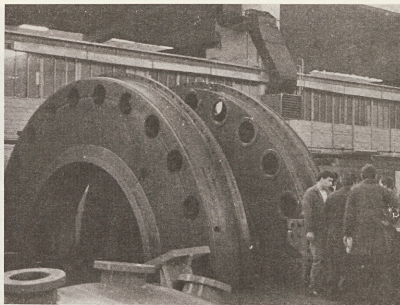
Obe polovici prvega turbinskega pokrova za Francisovo turbino za HE Stratos. Pokrov je pripravljen za transport po kopnem (ob izidu časopisa bo že prispel na gradbišče v Grčiji)
