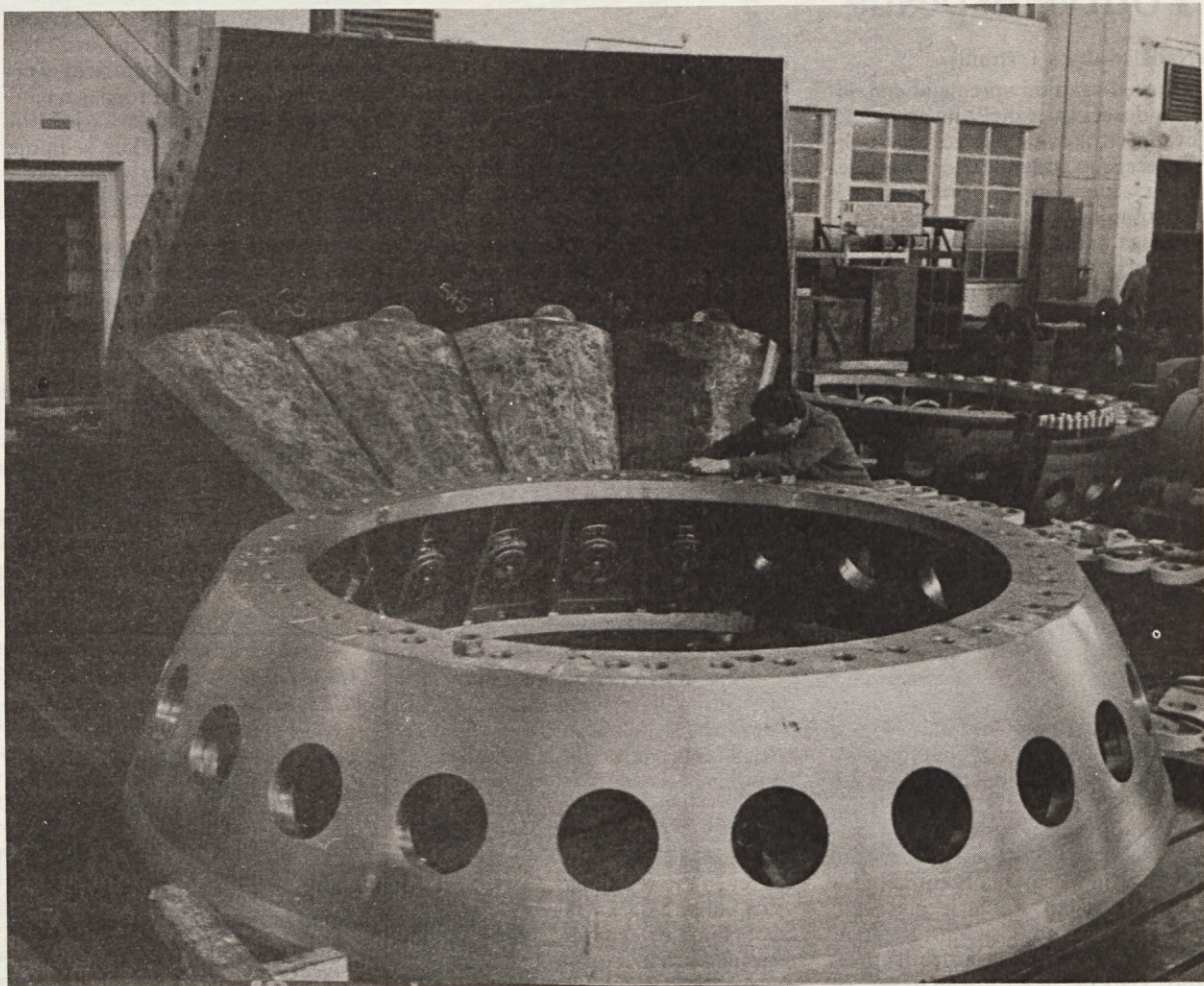
Prva poizkusna montaža koničnega vodilnika za cevno turbino za HE Dubrava (Foto: E. L.)
