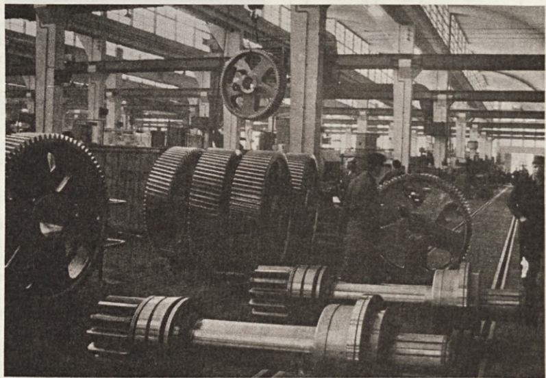
Priprava komponent za montažo bagerskih reduktorjev (Foto: E. L.)
