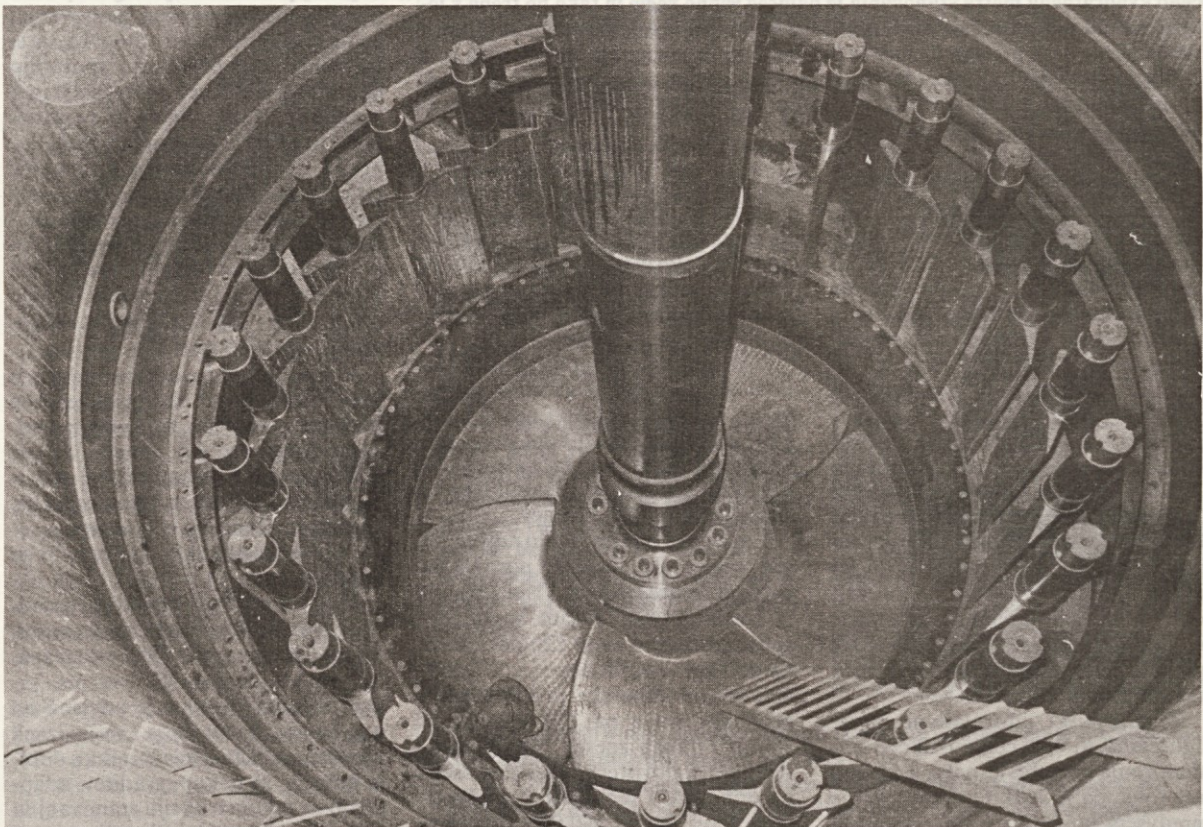
Pogled na vodilnik in gonilnik z gredjo med montažo
