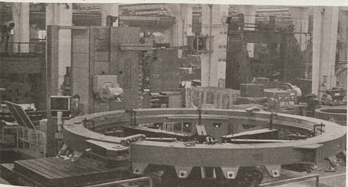
Regulirni obroč za HE Dubrava — obdelava izvrtin pod kotom na CNC stroju Colgar. Vrtanje in delitev izvrtin se izvaja s pomožno vrtljivo mizo, saj je premer obroča »samo« 9 metrov. Delo se izvaja na celotnem drugem polju (delno pa celo v prvem), tako da je zaprta tudi transportna pot. Ali bo potrebna za HE Vrhovo tudi takšna iznajdljivost, ali pa bomo morda lahko obdelovali v novi hali s primerno velikim strojem? (Foto: E. L.)
