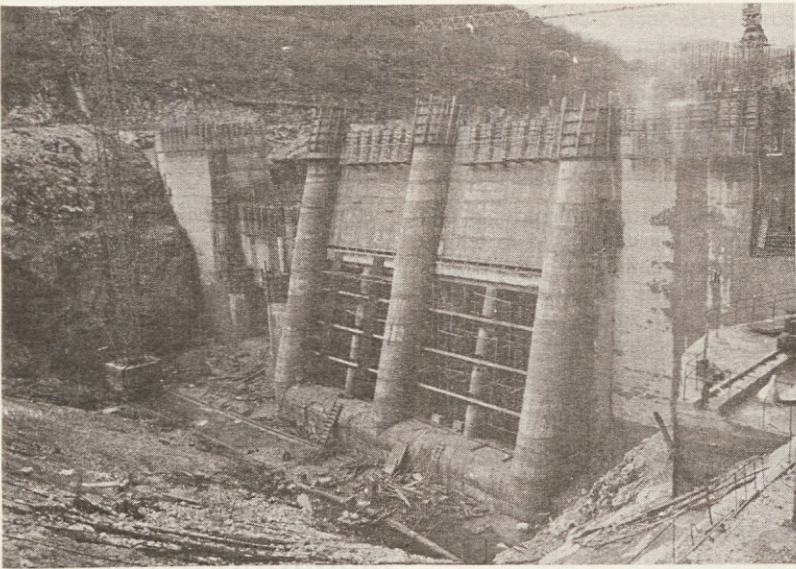
Že naslednje leto bo vstopni del elektrarne prekrivala voda akumulacijskega jezera
