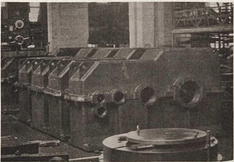
Vrtnanje izvrtin na AC-reduktorjih ter priprava na transport v montažo za junijsko realizacijo
