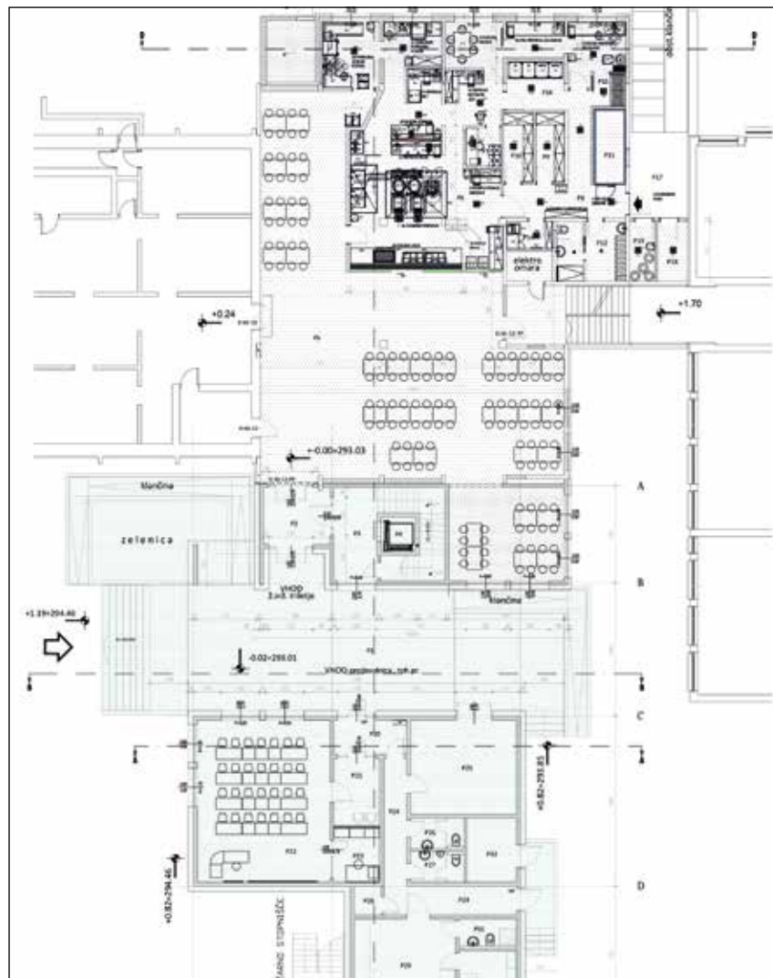
Izsek iz načrta: tloris pritličja
