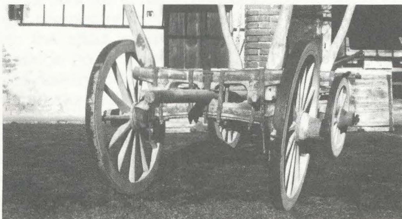
Zadnji del voza, v sredini gleda nazaj repica t.j. konec svore, ki povezuje sprednji in zadnji del, hkrati pa omogoča tudi različne razdalje med sprednjim in zadnjim delom voza
