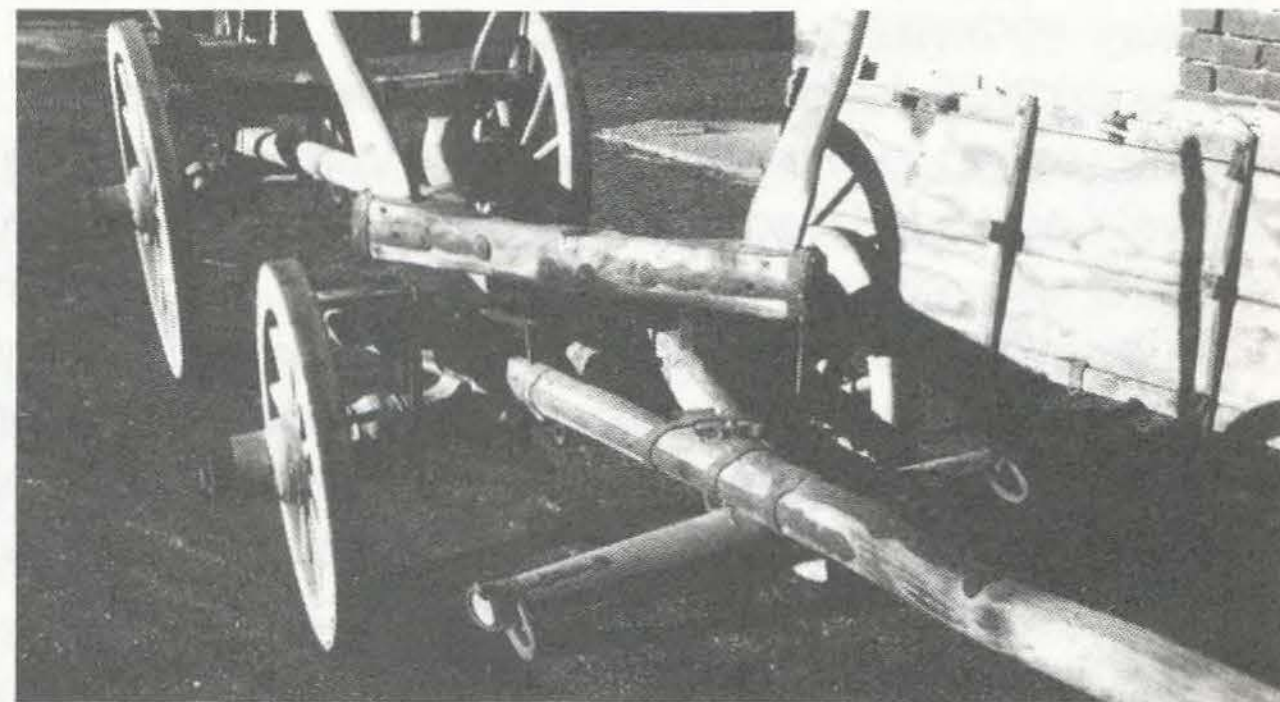
Voz brez poda- sprednji del z vrtelom in ročicami, po sredini svora, na katero so zadaj pritrjene trabi t.j. del zadnje osovine
