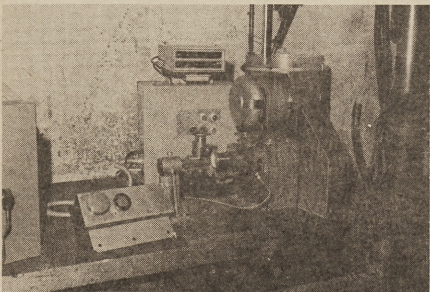
Navijalni stroj – „domać“ izdelek v Elektromotorjih.
