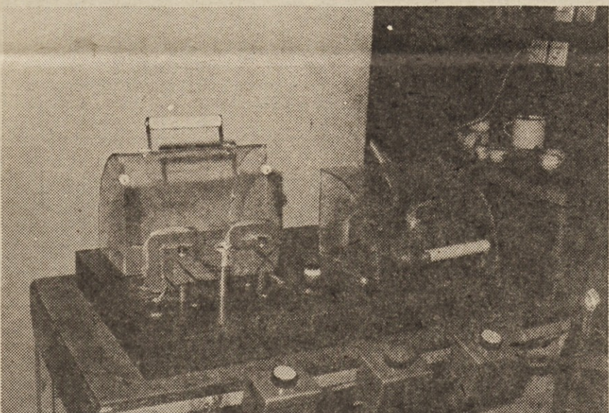
Naprava za magnetenje permanentnega magneta.
