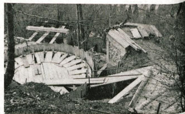
Gradnja 100-kubičnega vodnega rezervoarja je težavno in zahtevno delo, kajti zaradi nedostopnega terena, vsa dela potekajo ročno.
