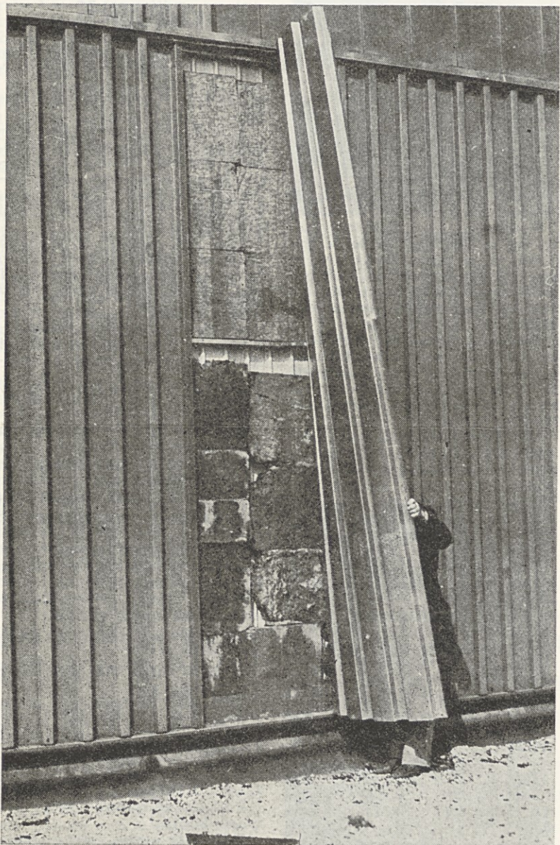
Izredno pomanjkljivo položena izolacija na valoviti strehi prizidka PS V
