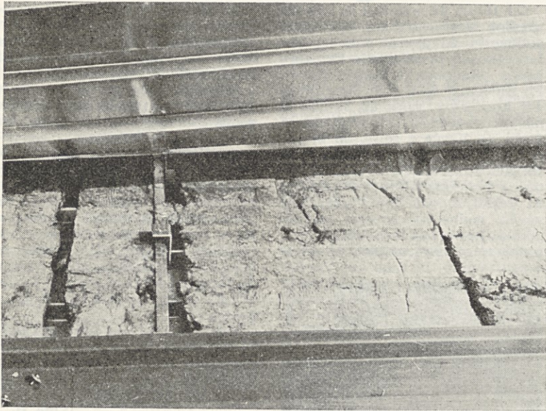
Izredno pomanjkljivo položena izolacija na valoviti strehi prizidka PS V
