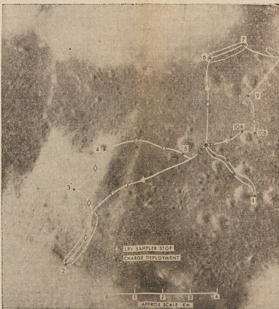
POTOVANJA CERNANA IN SCHMITTA PO LUNI — Na fotografiji Lunine površine so zaznamovana tri potovanja astronautov E. Cernana in H. Schmitta po Lunini površini. Prvo s št. 1 na koncu je bilo opravljeno v ponedeljek ponoči in v prvih urah torka. Sinoči sta šla astronauta na pot, ki je dosegla največjo oddaljenost od njunega oporišča v lunski ladji pri št. 2. Danes bosta opravila zadnje potovanje, nato pa pregledala vse opravljeno in nabrano, predno se bosta jutri zvečer dvignila z Lune na pot proti domu.
