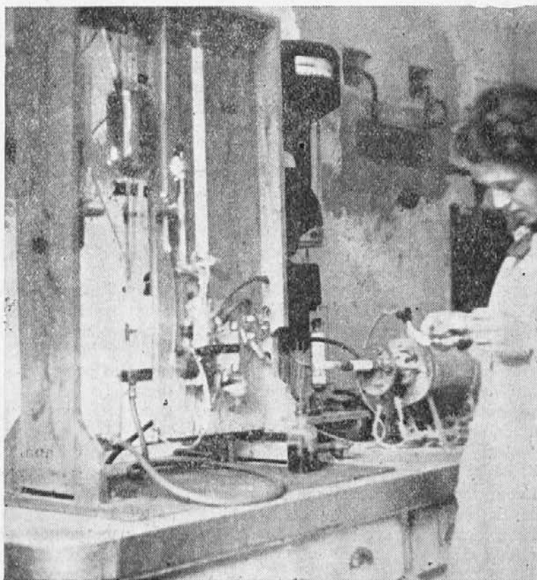
Aparat za določanje ogljika in žvepla.
