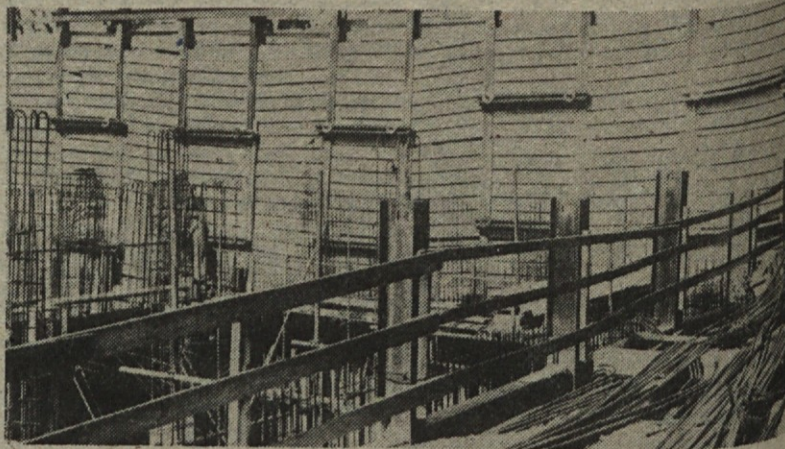
Navpični izkop, zavarovan z berlinsko steno
