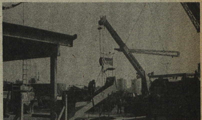
Za postavitev, oz. demontažo sejemskih eksponatov so nujno potrebna tudi avtodvigala
