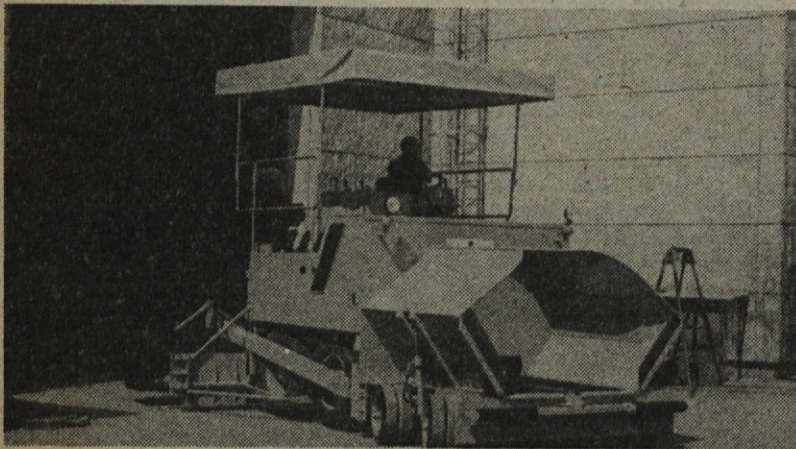
Finiŝer K-6 je zapeljal iz proizvodne hale
