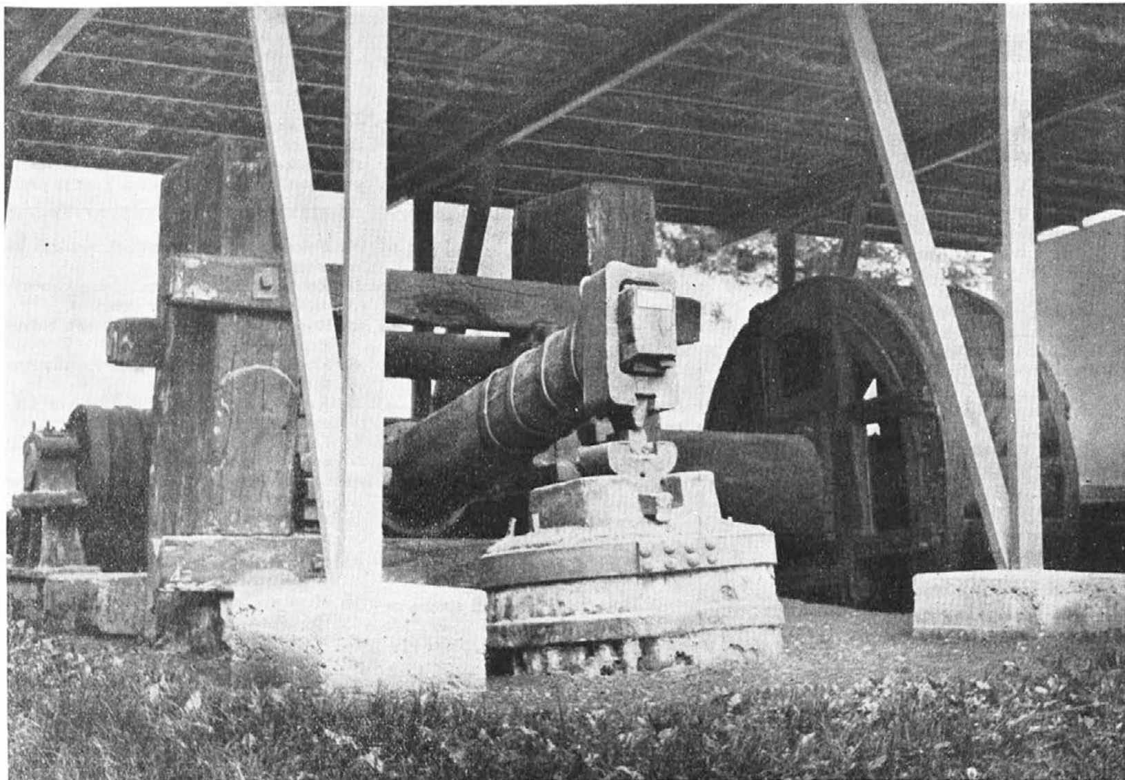
Repač — zmerom bolj smo ponosni nanj — na ta prvi zunanji objekt v našem muzeju. Tradicija kovačij ob naših vodah je v njem in svojsvena tehniška pogruntacija. Železarji so ga pokrili, da ga ohranimo rodovom za nami
