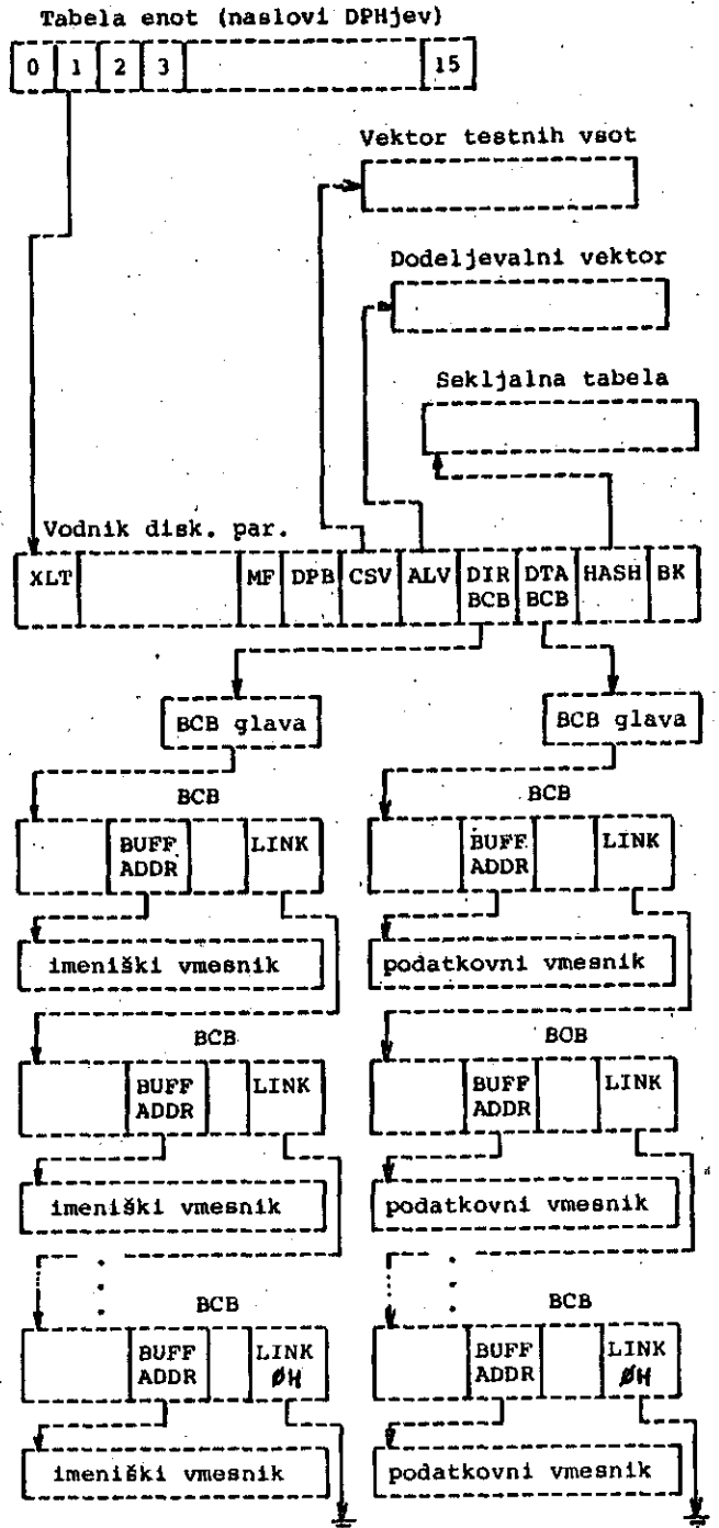
Slika 1. Bančni sistem BIOS podatkovnih struktur v sistemu CP/M Plus
