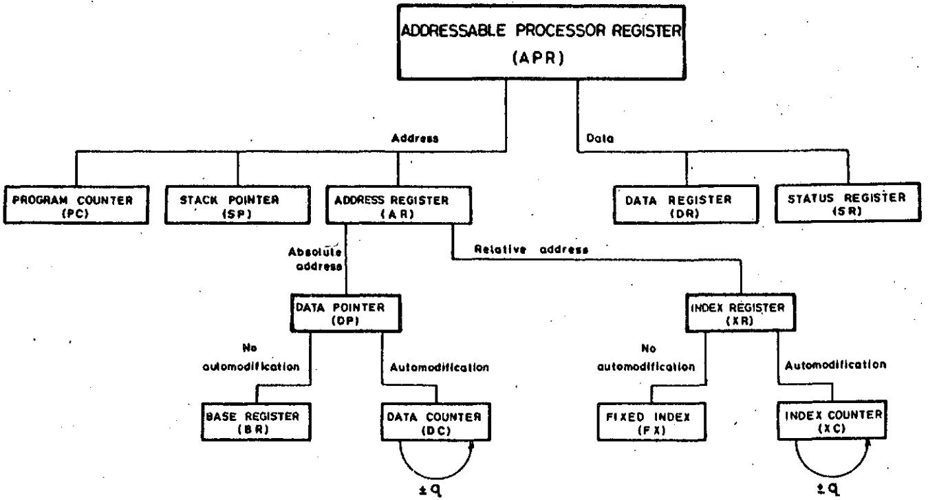
Slika 1. Klasifikacija adresabilnih procesorskih registara
