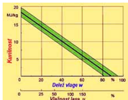
Odvisnost kurilnosti v MJ/kg od deleža vlage v drveh in vlažnosti drv (Vir: TFZ Bayern)
