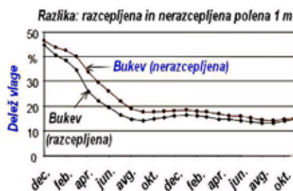
Zniževanje vlažnosti bukovih razcepljenih in nerazcepljenih drv v obdobju dveh let (Vir: TFZ Bayern)
