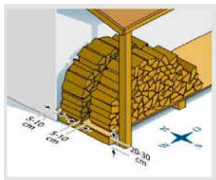
Nasekana drva sušiti zložena in z naravnim prezračevanjem, pokrita proti dežju, na sončni strani (Vir: www.bosy-online.de)
