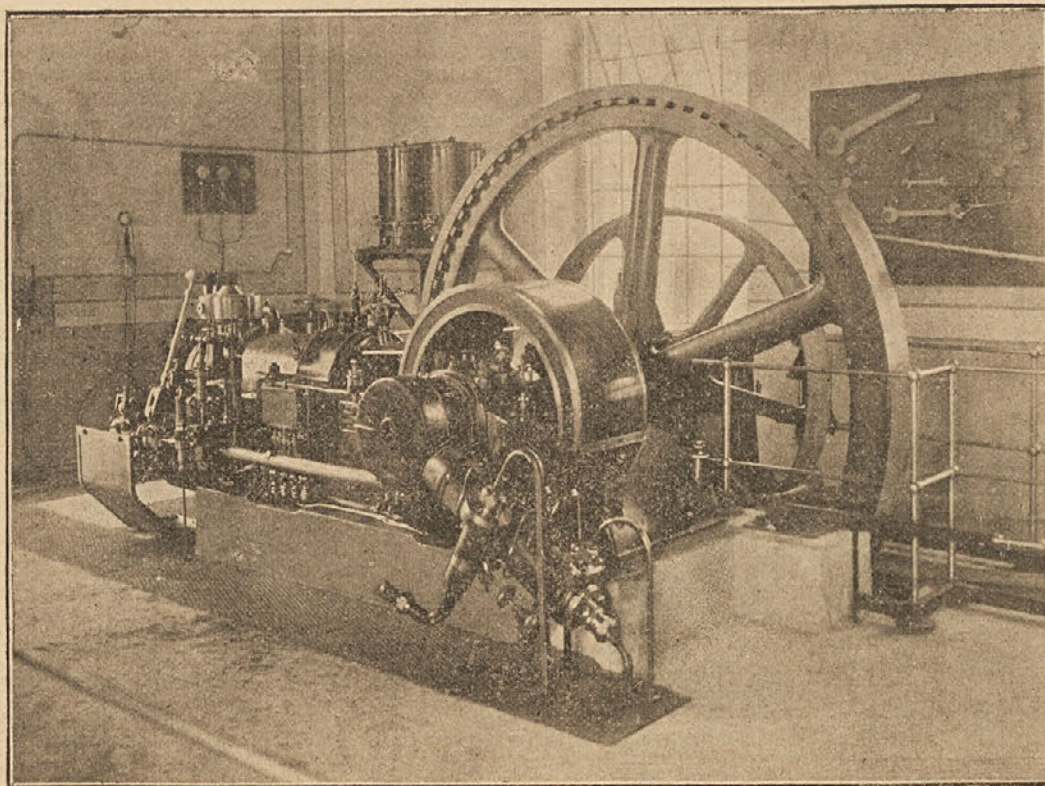
Iz „Zadružne elektrarne“ v Trbovljah: glavni stroj.
