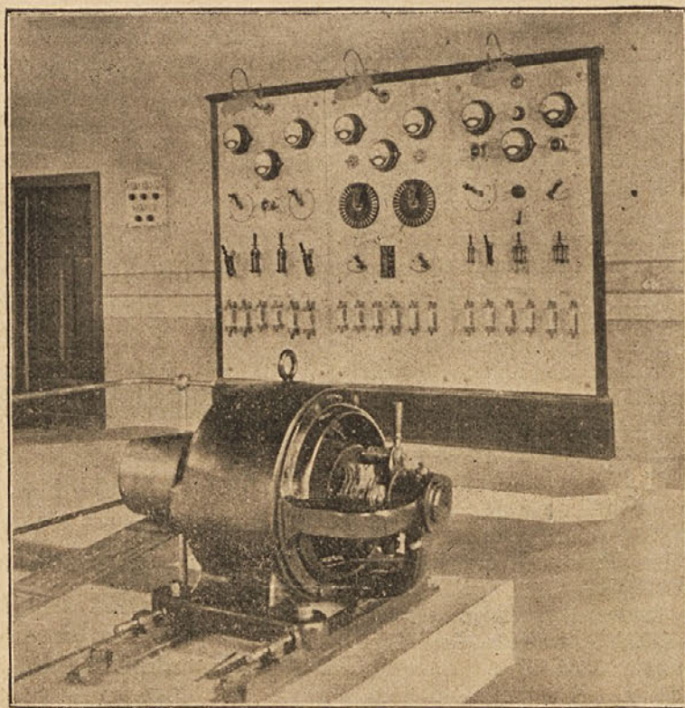
Iz „Zadružne elektrarne“ v Trbovljah: dinamostroj.
