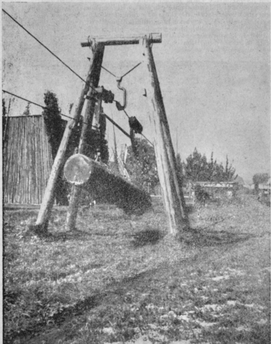
Takle težak hlod iz vsake grape potegne na vozno pot najbolje le žičnica. Koliko prihranjenega truda, znoja in nesreč. Les pa pride nepoškodovan do kupca in krajev, kjer ga predelujejo.
