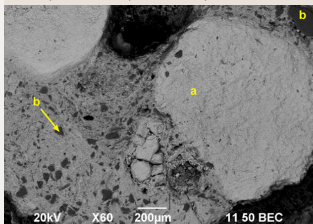
48 Iz SEM posnetka je razvidna slaba sortiranost vzorca. Pogosta so velika zaobljena zrna Fe-oksida (a) in manjša zrna kremena (b). Pod sliko sta EDS spektra Fe-oksida (sp. 1) in kremena (sp. 2).
