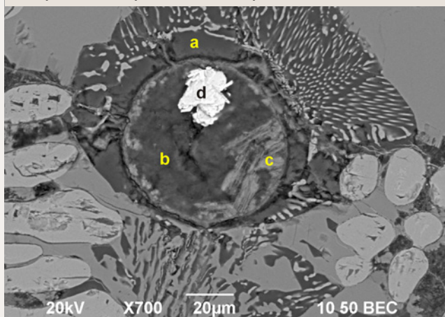
46 Kroglasti vključek v levcitni osnovi (a), zapolnjen z almandinom (b), igličastimi kristali Fe-oksida (c) in zrnem barita (d). Pod sliko sta EDS spektra barita (sp. 1) in almandina (sp. 2).
