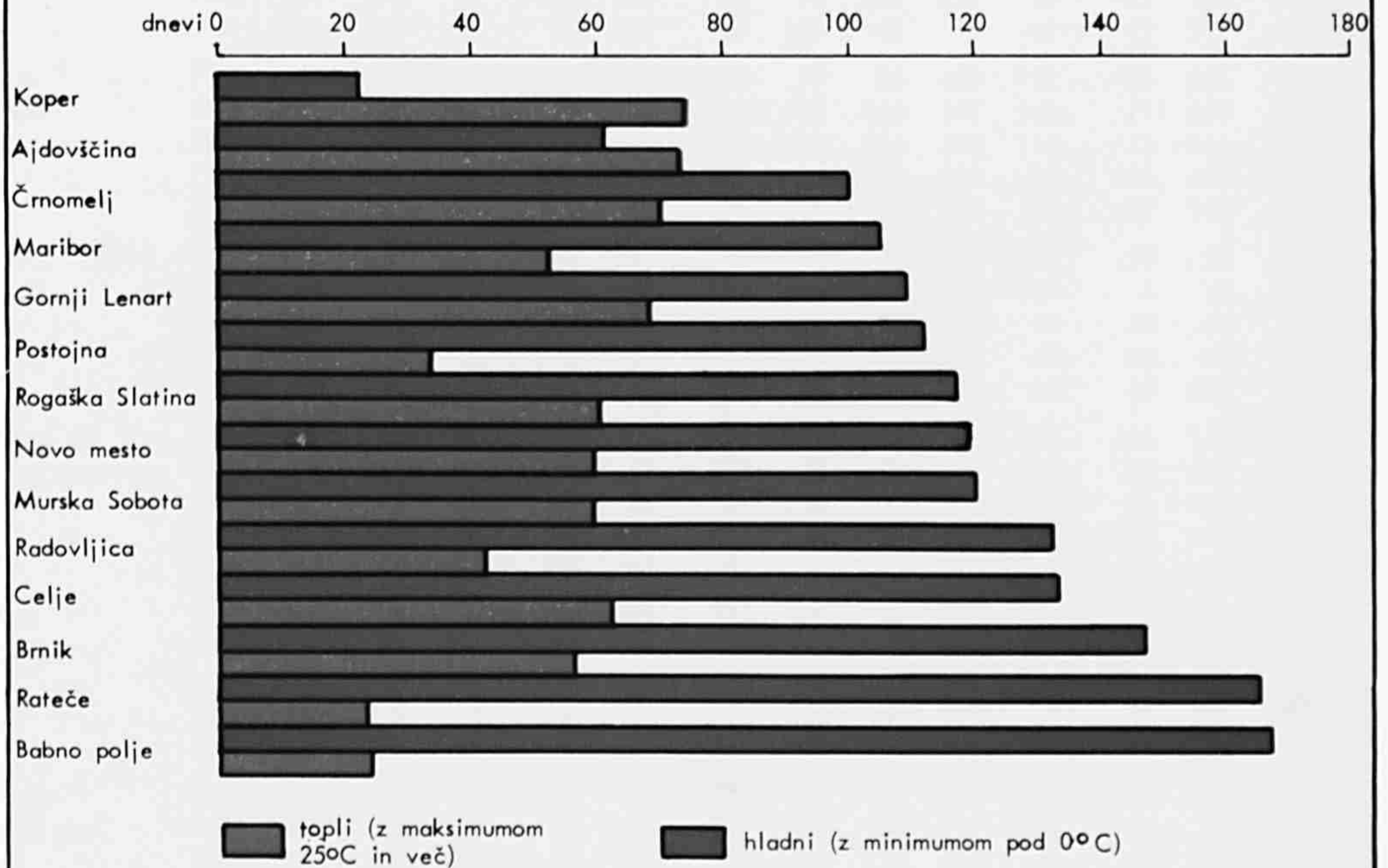
Topli in hladni dnevi (letno poprečje 1967 - 1971)
