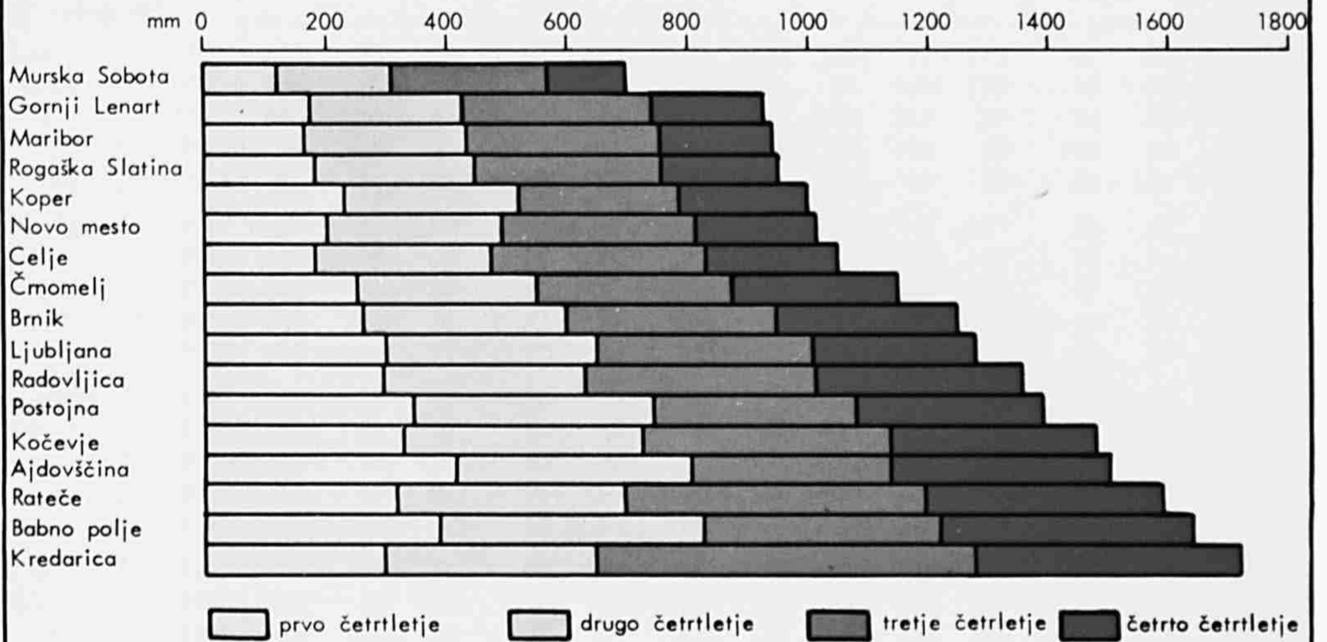
Letna in četrtletna višina padavin (poprečje 1967 - 1971)
