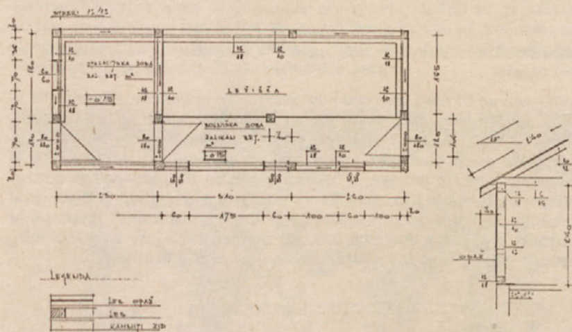
Skica prostora za ranjence in razkuževalnice z izmerami; doris
