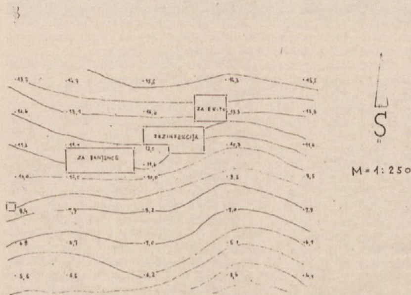
Skica kraja, kjer so bili postavljeni objekti bolnice „Jesen“, na terenu z vrisanimi plastnicami;
