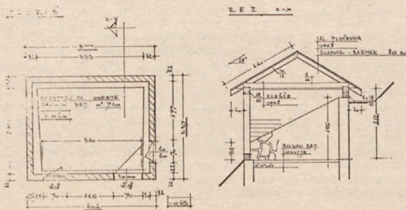
Skica objekta za osebje bolnice „Jesen“ z izmerami; tloris prostora in rez x-x objekta
