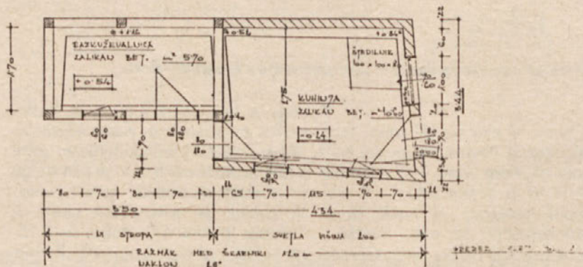
Skica kuhinje in razkuževalnice z izmerami; tloris (prerez glej rez na strani...)
