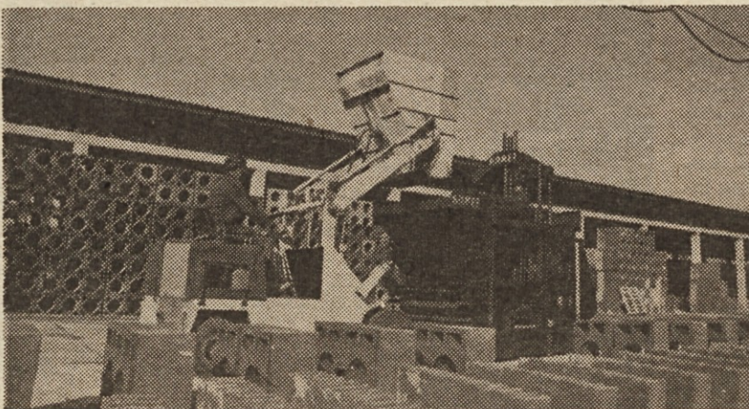
Stroj za izdelovanje dimnih tuljav je pravzaprav podoben finišeju, ki polaga asfalt, le da za tem strojem ostajajo elementi za dimne tuljave
