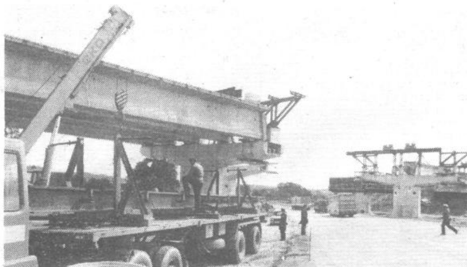
Spet en posnetek z gradbišča zahodne obvoznice. Nadvoz pri Dolgem mostu bo kmalu sklenjen. Po novi obvoznici pa bo stekel promet že septembra.
