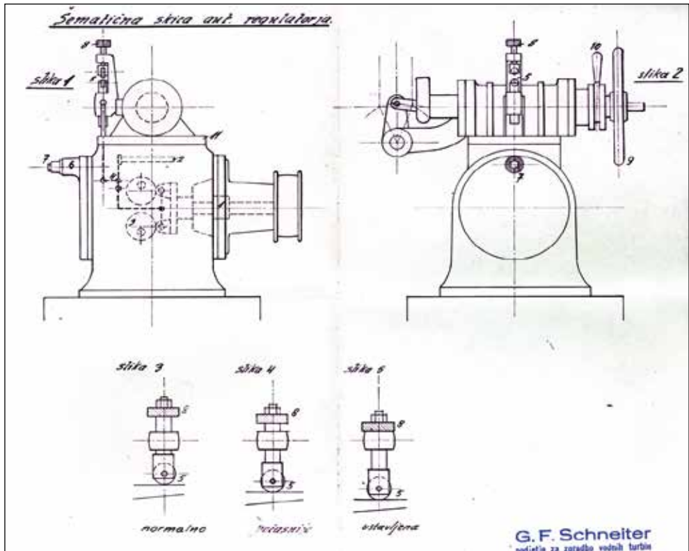
Shematična skica avtomatskega regulatorja podjetja G. F. Schneiter.
