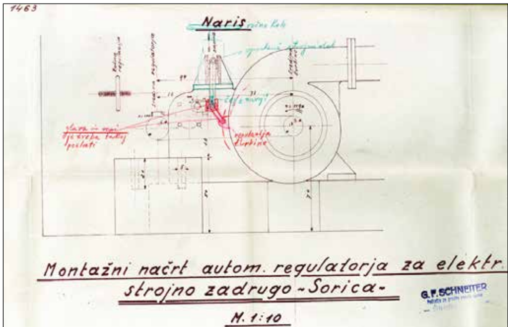
Načrt za montažo avtomatskega regulatorja podjetja G. F. Schneiter iz Škofje Loke, poleti 1939.
