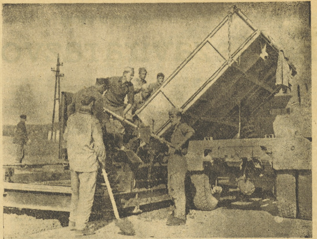
Devetkratna udarna karlovska mladinska delovna brigada se je posebej usposobila za betoniranje cestišča. Vrsta mladincev se je naučila ravnanja z gradbenimi stroji. Tej brigadi je pripadla tudi čast, da so zabetonirali zadnji meter avtomobilske ceste. — Na sliki: betonsko mešanico stresajo s tovornjaka v razdelilec.
