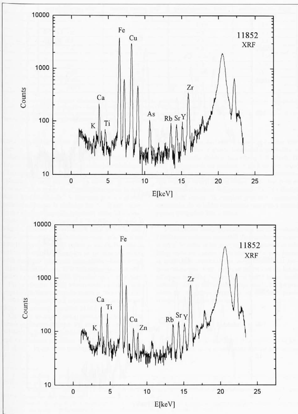
Sl. 1: Rentgenski spekter notranje (zgoraj) in zunanje površine (spodaj) največjega kosa predmeta 11852, izmerjen z metodo rentgenske fluorescenca (XRF).
