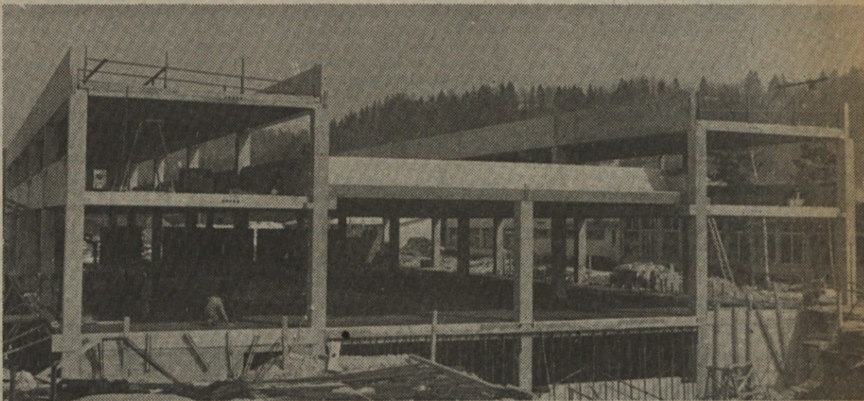
Nova proizvodna hala za Iskra Otoče je dolga 50 in široka 30 metrov. Postavili so jo delavci tozda OGP, njena specifičnost pa je šedova streha
