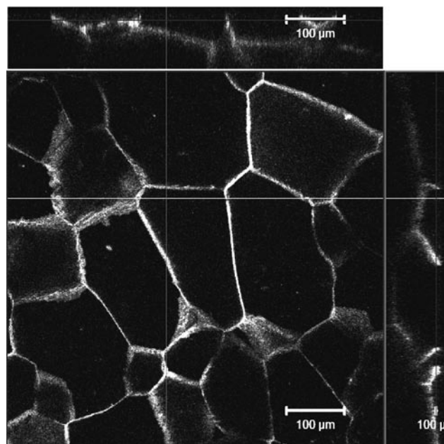
Slika 6. Posnetek toplotno staranega marmorja po 50 ciklusih ogrevanja in ohlajanja v temperaturnem razponu od 20 do ca. 60 °C. Na sliki je vidna jasna mreža razpok med zrni, ki se nadaljujejo tudi v globino (povečava objektiva 20 \times ; 0,75 NA, globina posnetka je 82 µm)
