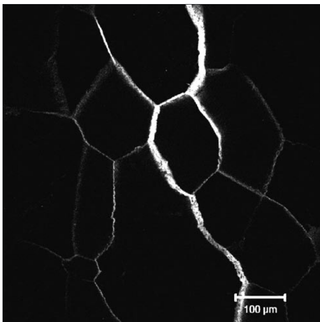
Slika 5. Mreža trans-granularnih razpok v toplotno staranem marmorju (povečava objektiva 20 \times ; 0,75 NA)
