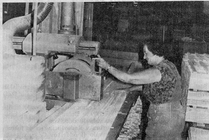
Narez pokončnikov za B 4
