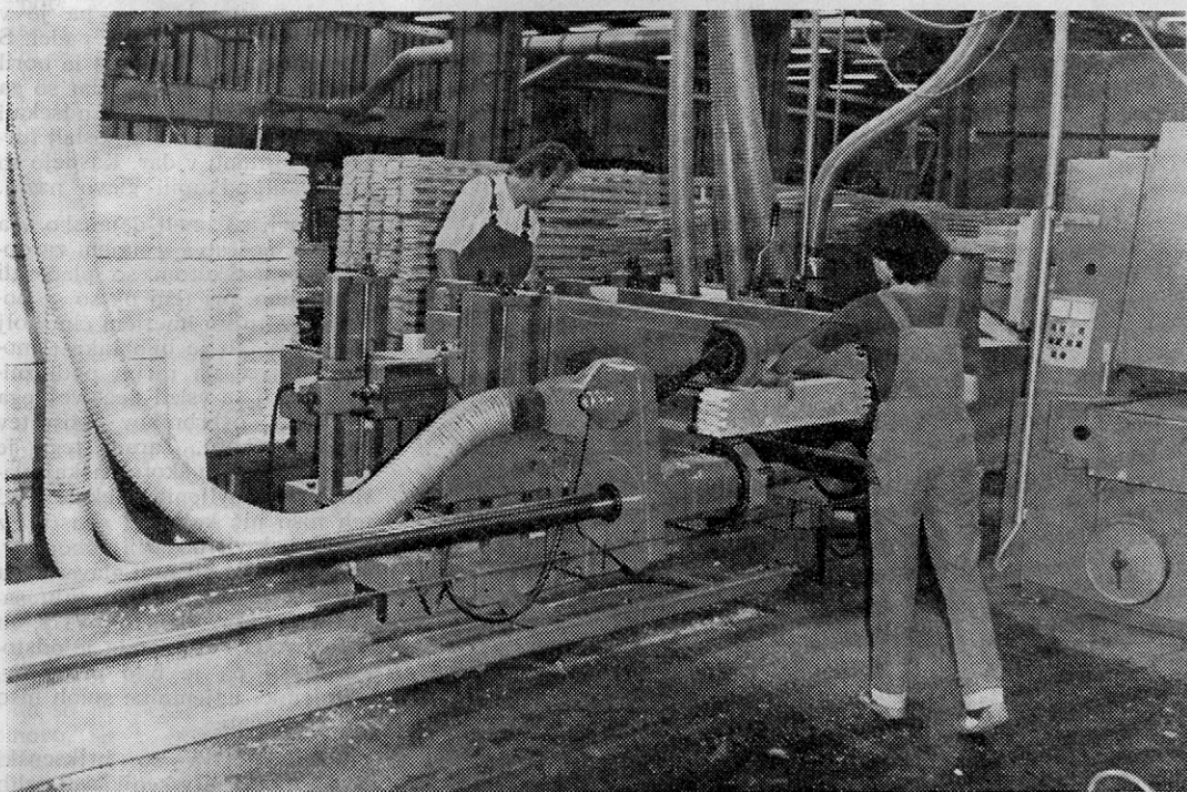
Rogličenje in brušenje podbojev B4
