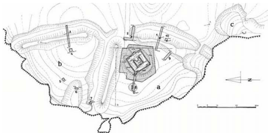
Tloris gradišča nad Pivko pri Naklu (VALIČ, 1968). The groundplan of an ancient fort above Pivka near Naklo (VALIČ, 1968).
