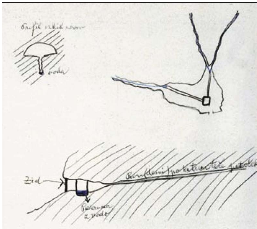
Pretmerjeva skica jame Velika Lebinca iz leta 1946 (Kataster jam).
