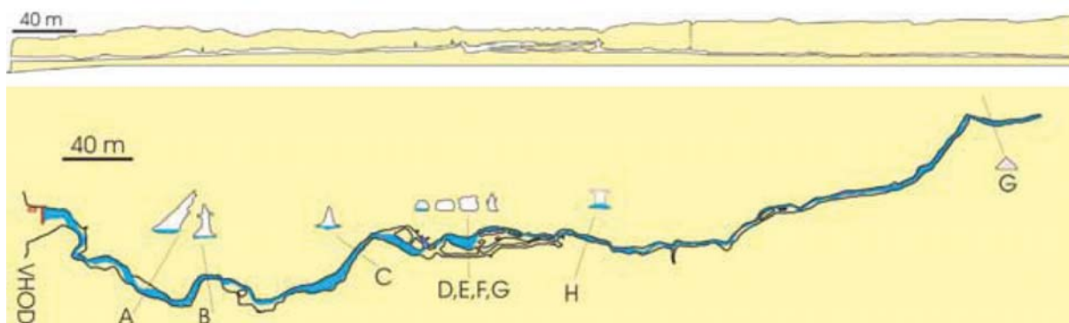
Tloris in profil Arneševe luknje (prirejeno po Gantarju (1955)).
