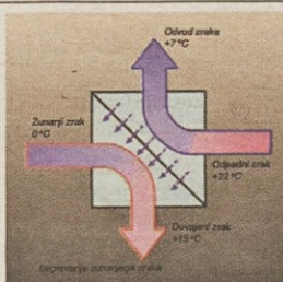
Skica 1: Osnovni princip delovanja rekuperatorja. Vir: internet
