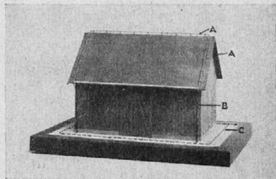
a lovilna napeljava, b odvodna napeljava, c ozemljevalna napeljava.
