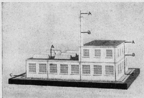
a lovilna napeljava, b odvodna napeljava, c ozemljevalna napeljava.
