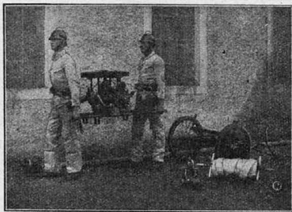
Prenosna lahka motorna brizgalnica (agregat, ki ga neseta dva gasilca).
