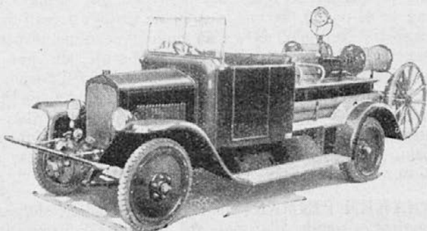
Podeželna automotorka s črpalko spredaj.
