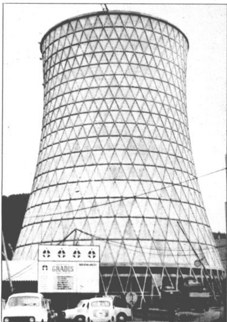
Ponos delavcev Gradis – TOZD Gradbena enota Celje je tudi hladilni stolp šoštanske velikanke – TEŠ 4
