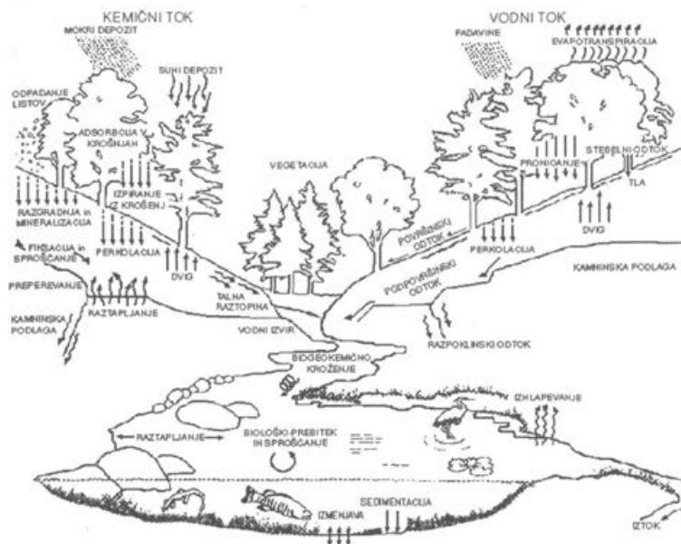
Slika 1. Kroženje vode na gozdnatem zemljišču (Johnson & Van Hook, 1989).
