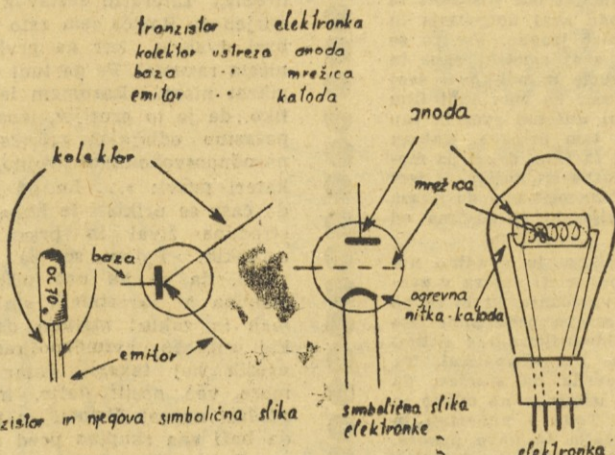
SL.1. Primerjava elektronke s tranzistorjem
