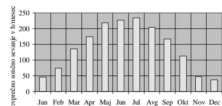
Diagram: Porazdelitev sončnih ur na mesec
