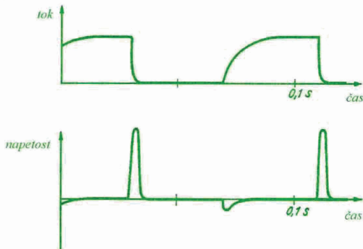
Slika 5. Časovna odvisnost toka po krogu s prekinjalom v induktorju (zgoraj) in sunki inducirane napetosti na cevi (spodaj).
