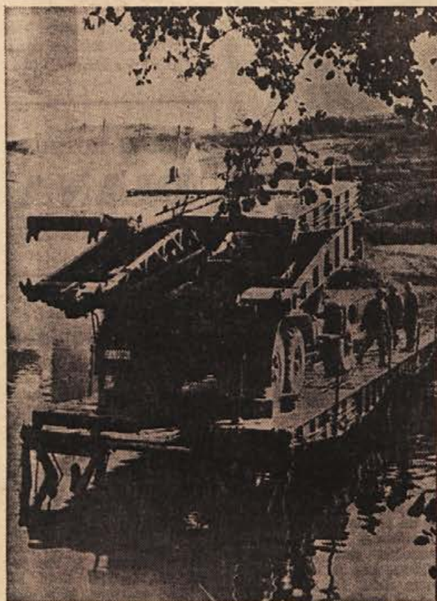
Pretekli četrtek so enote JLA v okviru vojaških vaj preizkušale sodobno orožje in opremo. Preko reke Dobre na Hrvaškem so v manj kot poldrugi uri postavili montažen most, preko katerega gredo lahko tudi najtežja vojaška vozila. (Foto: Ria Bačer)
