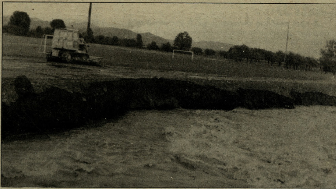
Voda je odnesla in razdejala del nasipa na reguliranem delu Bolske.
