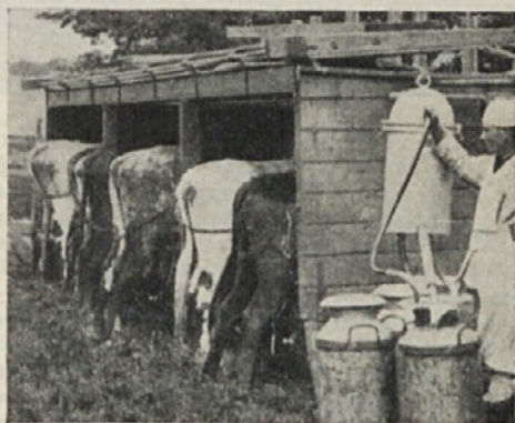
Šest krav je mogoče naenkrat molsti. Mleko teče v odvajalne cevi in odtod v zbiralne posode.
