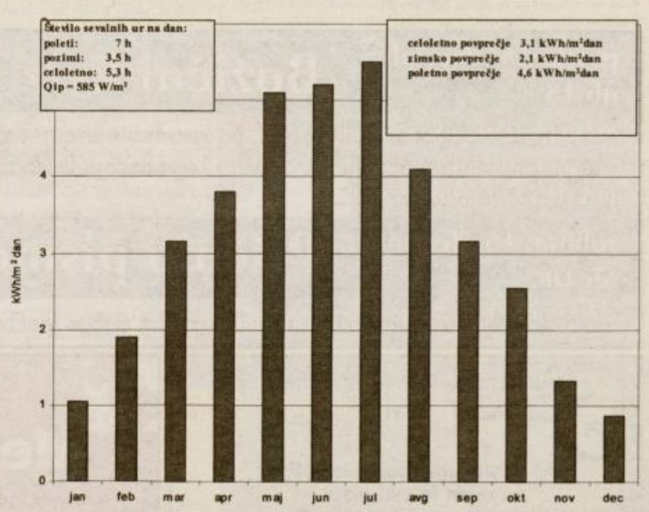
Sončno dnevno globalno sevanje na horizontalno ploskev (kWh/m 2 dan)
