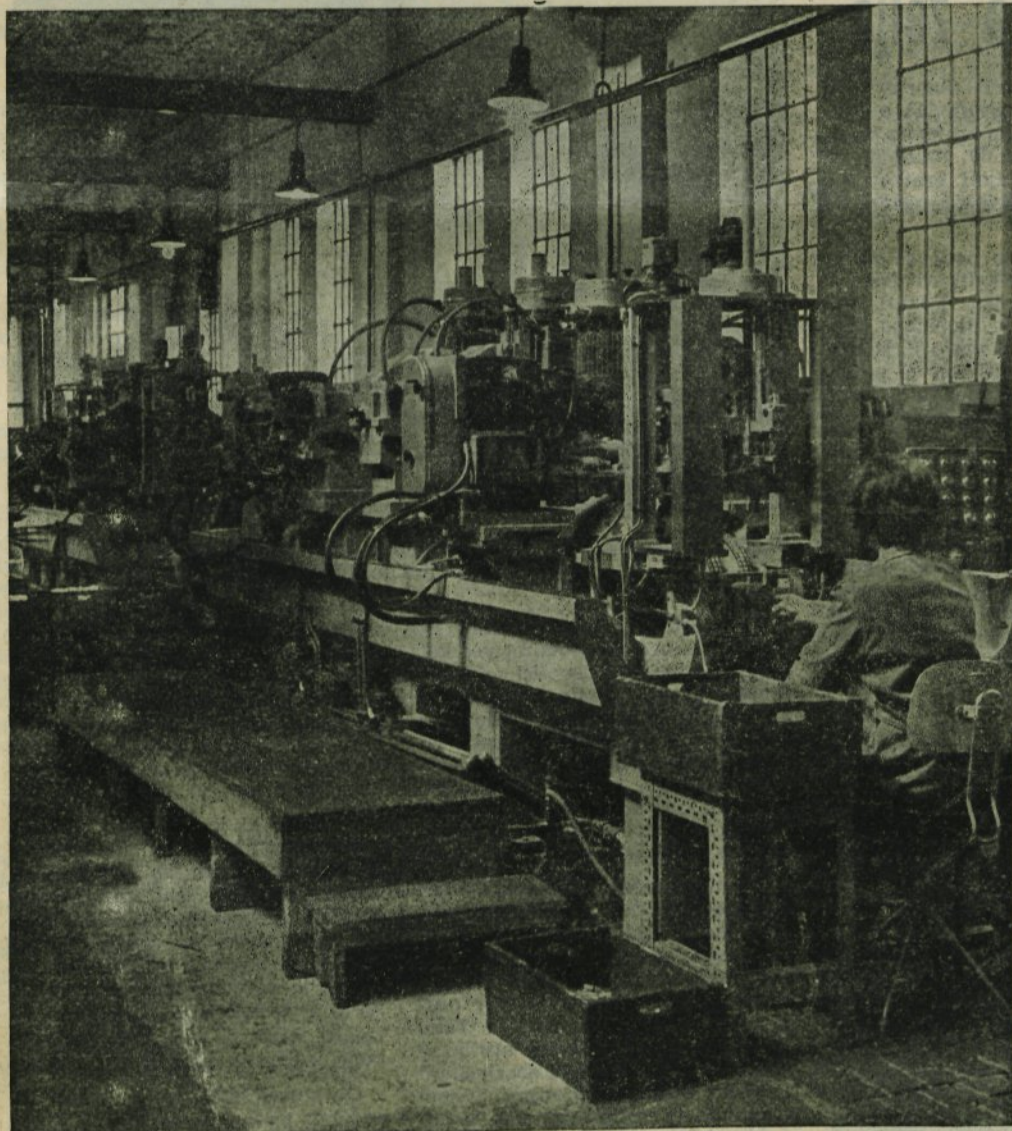
Transferna proga za obdelavo cilindrov.
